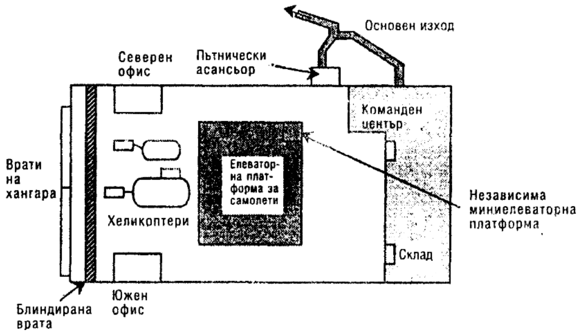
НИВО 1: ХАНГАР
